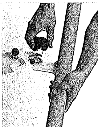
Particolare della regolazione in larghezza del corrimano.
