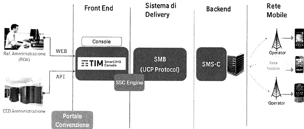
Figura 3 – Architettura applicativa della piattaforma SMS massivi.
