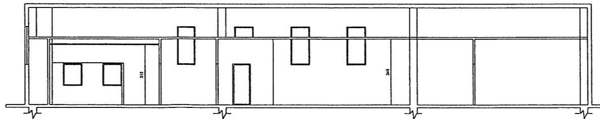
SEZIONE B-B - SCALA 1:50
